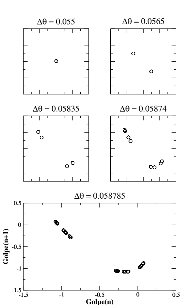
Figura 6. Primer mapa de retorno para las fases donde golpes sucesivos sincronizan. Los ejes son los mismos para todos los gráficos, mostrado en la parte inferior que corresponde al comienzo del caos.
